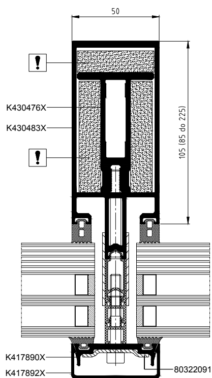
Przekrój przez słup EI 15, EI 30
