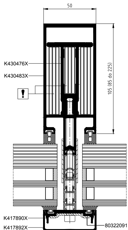
Przekrój przez słup EI 45, EI 60
